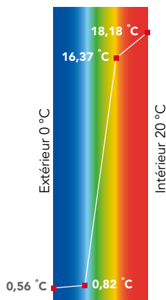
Évolution de la température mur creux avec 50 mm de laine soufflée
