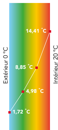
Évolution de la température mur creux non isolé
