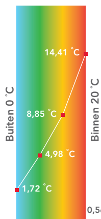
Temperatuurverloop ongeïsoleerde spouwmuur
